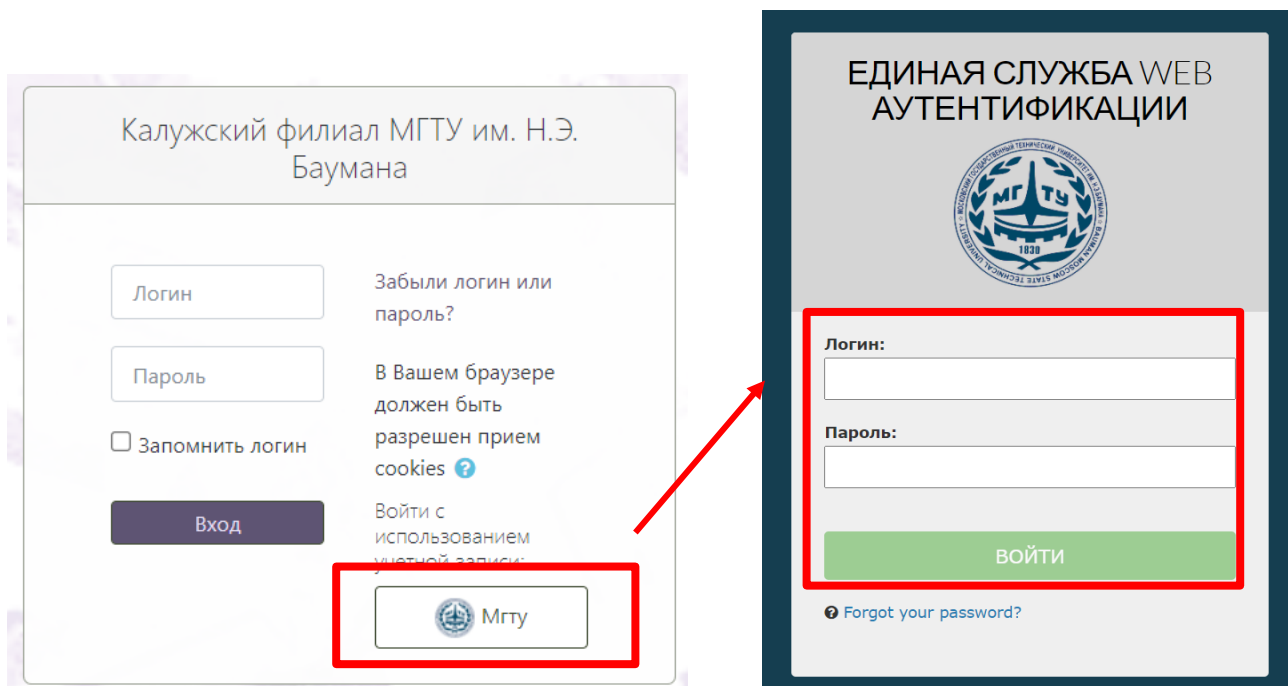
Рисунок 2. Окно аутентификации
